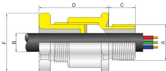
Cable wiring
